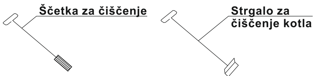
Slika 7. Oprema za čiščenje kotla BIO-PEK B
