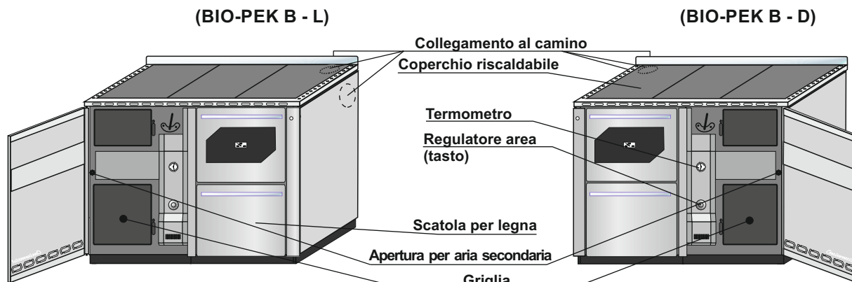
Foto 9. Componente generali
