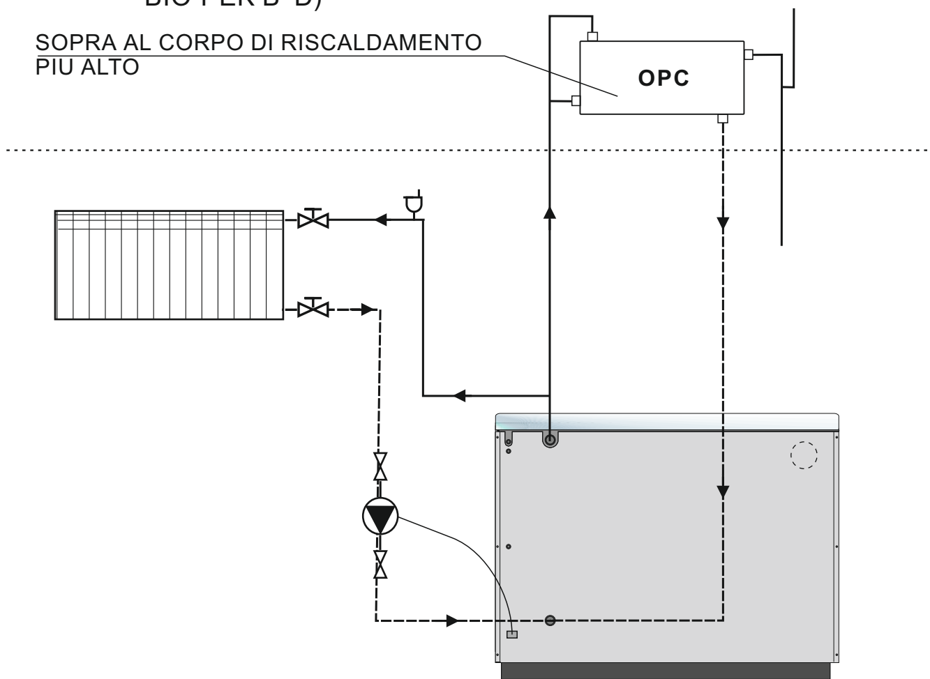
Schema 1: Collegamento della caldaia BIO-PEK B-L (vale anche per la caldaia BIO-PEK B-D)
