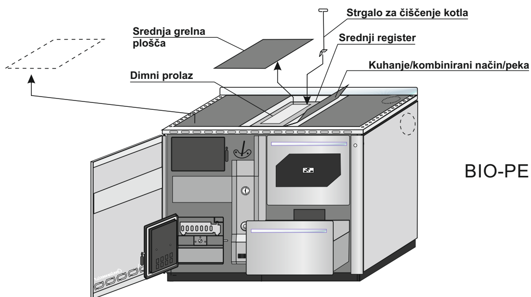
Slika 8. Čiščenje površin – kotel BIO-PEK B–D (velja tudi za kotel BIO-PEK B–L)
