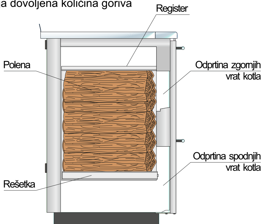
Slika 2. Najvišja dovoljena količina goriva
