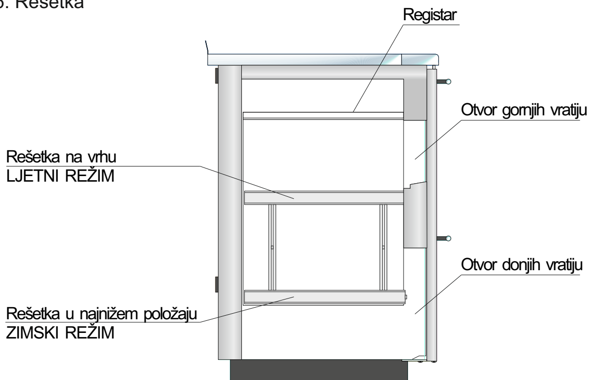
Slika 6. Rešetka
