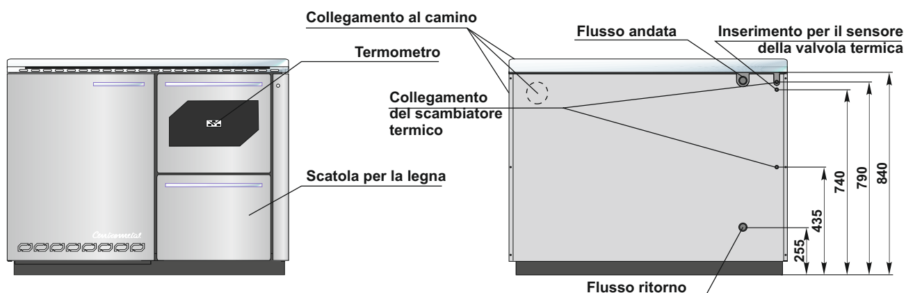
Foto 10. Caldaia BIO-PEK B – D (vale anche per BIO-PEK B – L)
