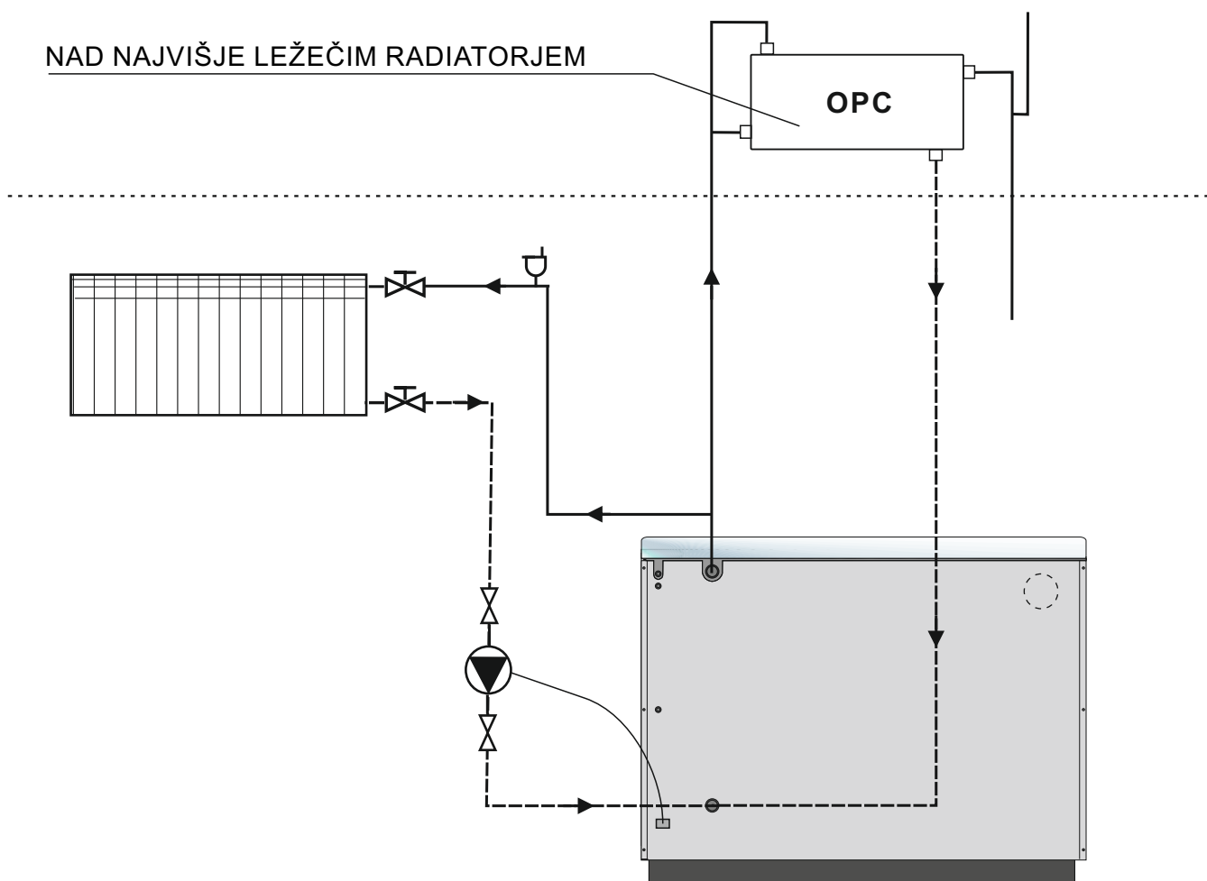
Diagram 1: Priključitev kotla BIO-PEK B–L (velja tudi za kotel BIO-PEK B–D)
