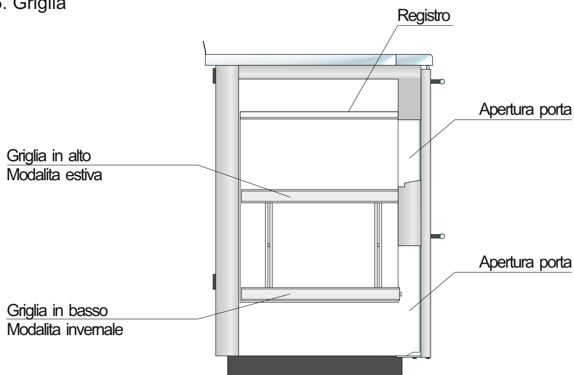
Foto 6. Griglia
