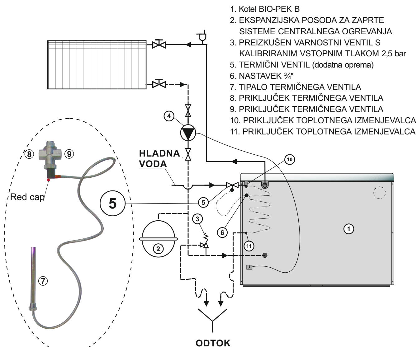
Diagram 2. Priključki kotla BIO-PEK B–L (velja tudi za kotel BIO-PEK B–D)
