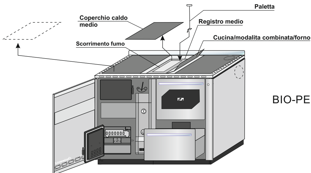
Foto 8. Pulizia – caldaia BIO-PEK B-D (vale anche BIO-PEK B-L)
