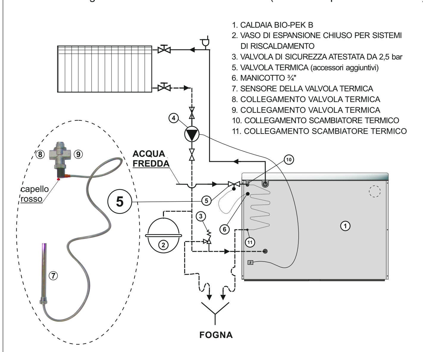
Schema 2. Collegamenti della caldaia BIO-PEK B-L (vale anche per BIO-PEK B-D)
