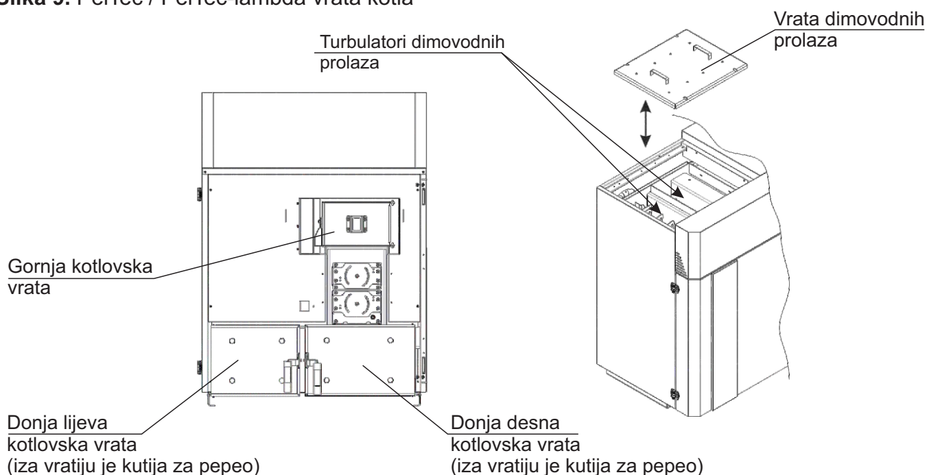
Slika 9. PelTec / PelTec-lambda vrata kotla
