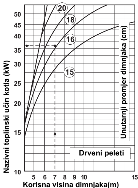
Slika 6. Dimenzioniranje dimnjaka za PelTec / PelTec-lambda
