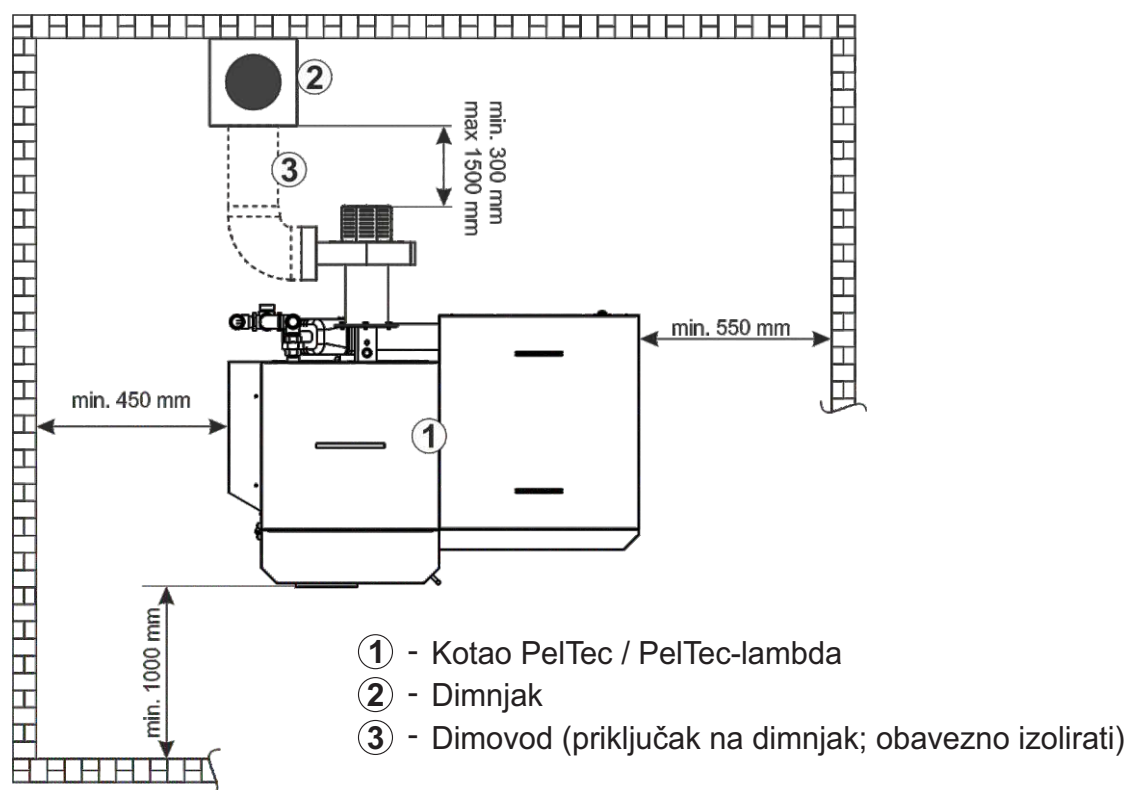
Slika 5. Minimalne udaljenosti od zida za PelTec / PelTec-lambda
