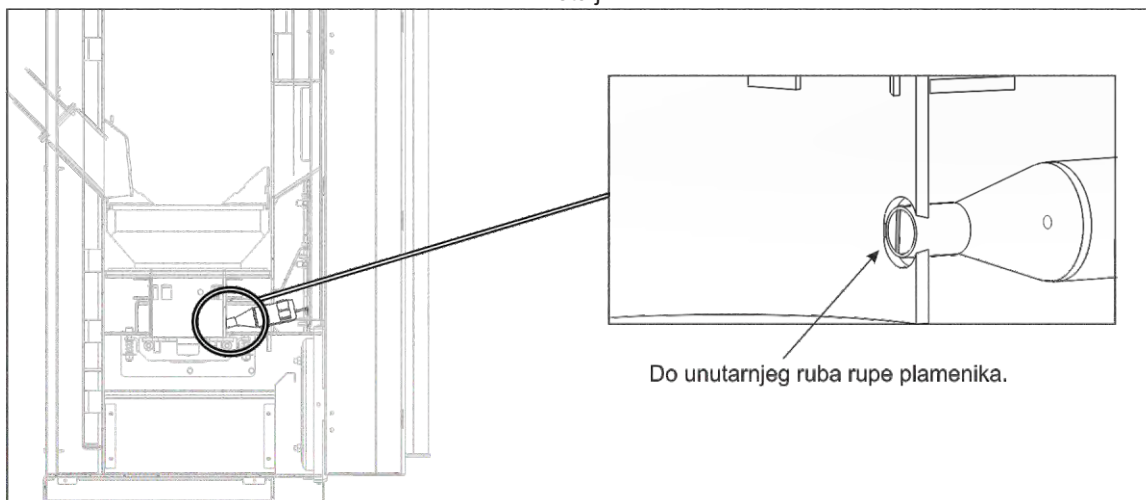
Detalj D
