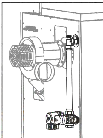
Primjer ugradnje pumpne grupe na kotao PelTec / PelTec-lambda 18-36
