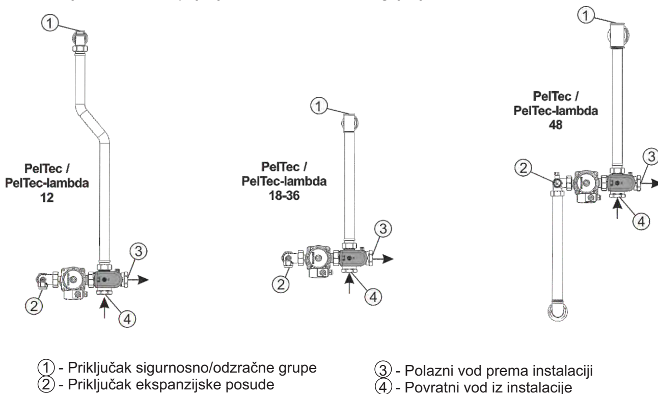
Slika 7. Priklučci kotla za spajanje na zatvoreni sustav grijanja
