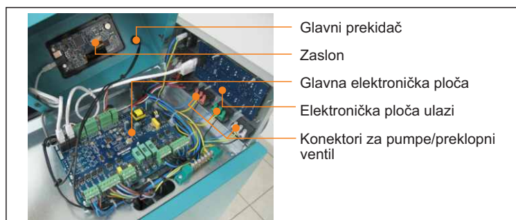
Slika 8. Konektori za priključenje napajanja, el. dijelova i osjetnika
