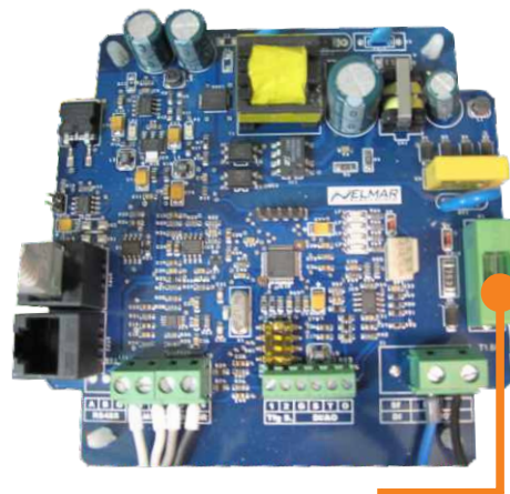
* Lambda štampana pločica (samo kod PelTec-lambda)
